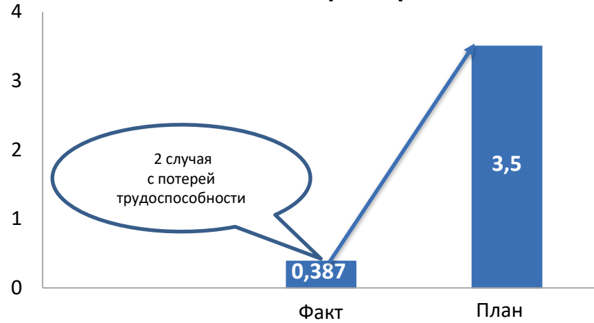
LTIF фактор
